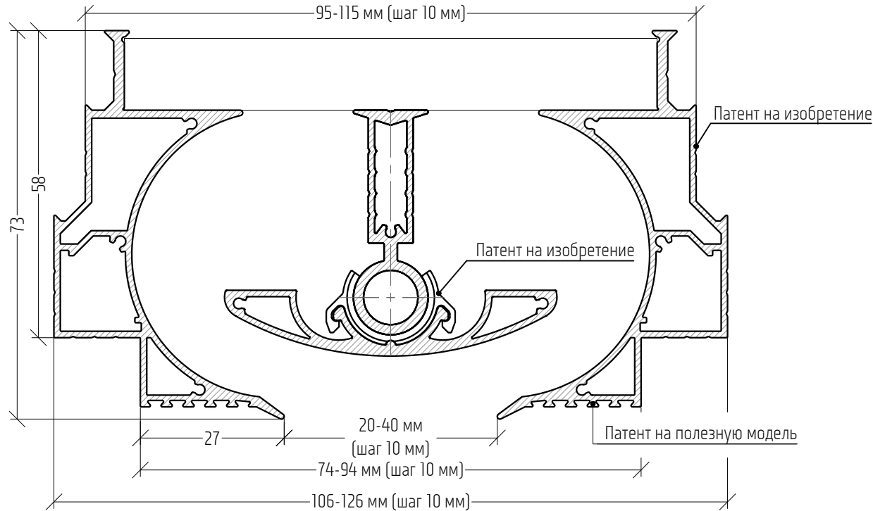
Сечение диффузора
